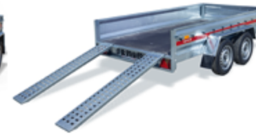
PRO 2612/2 • AUFFAHRRAMPEN AUS VERZINKTEM BLECH
