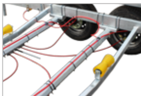
BREMSTROMMEL-SPÜLSYSTEM (ZUBEHÖR)
