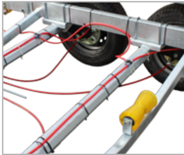
BREMSTROMMEL-SPÜLSYSTEM
