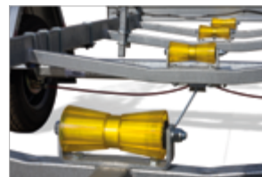
PROFILIERTE KIELROLLEN - für einfaches Zentrieren des Bootes, auch mit Höhenverstellung lieferbar
