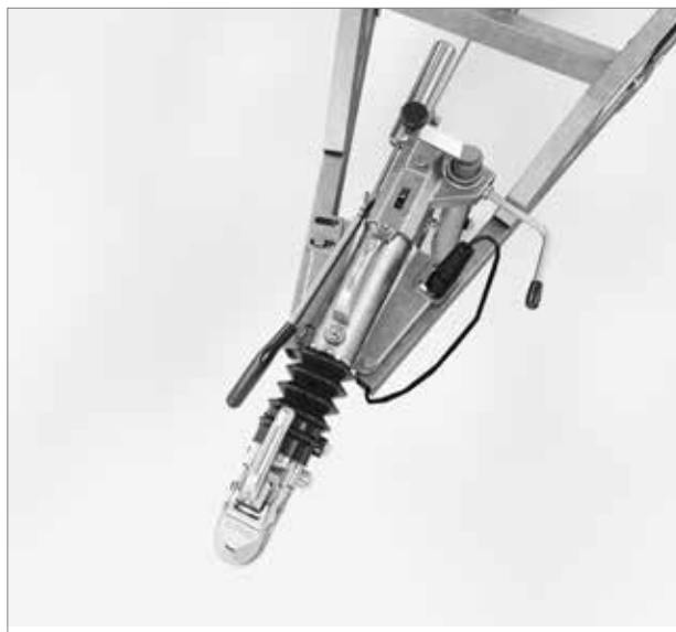
Durch die V-Deichsel, die bis zum Kugelkopf geht, erhalten Sie eine bessere Stabilität und ein ausgezeichnetes Fahrverhalten.
