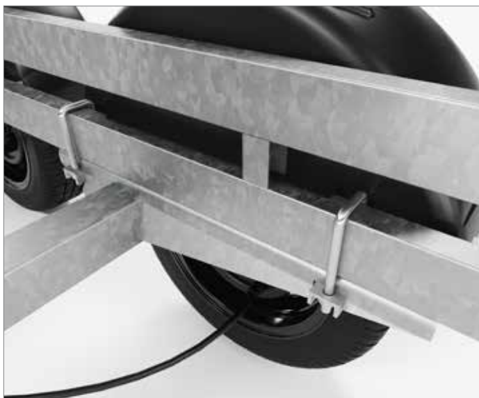
Verstellbare Achsen - die Achsen können individuell eingestellt werden um eine optimale Gewichtsverteilung und Stützlast zu erzielen.
